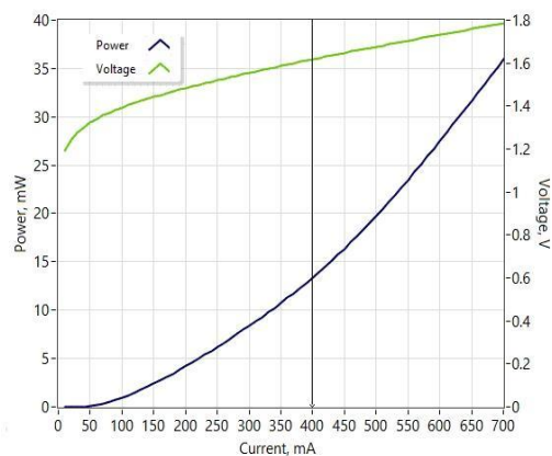
光-电流-电压特性
