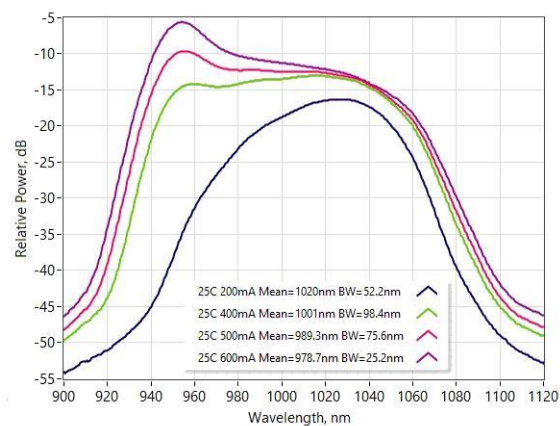
光谱 (分辨率 1nm)
