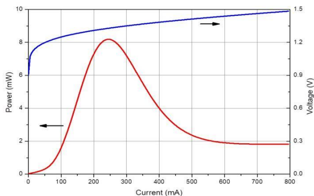
L-I-V 曲线
