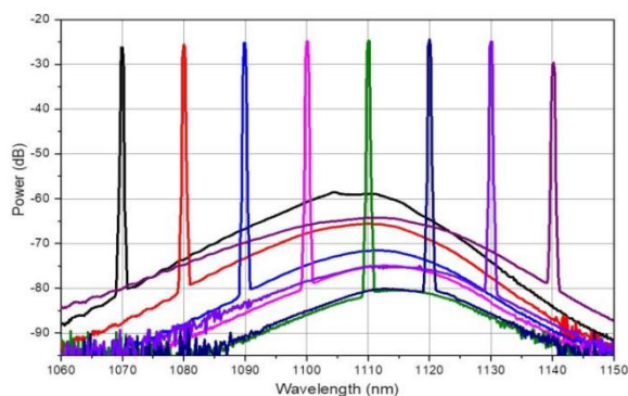
光谱(res. 0.5 nm)
