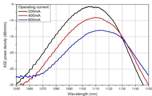
ASE 光谱 (分辨率 1nm)
