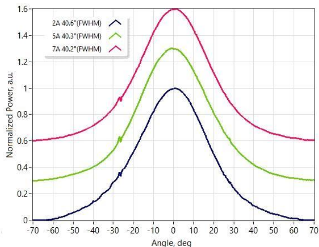
快轴远场
