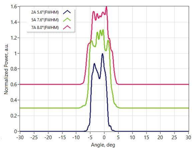
慢轴远场
