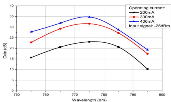
不同电流下的增益光谱
