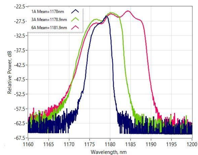
光谱（分辨率 1nm）
