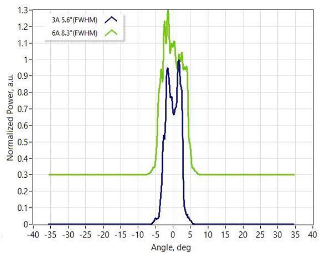
慢轴远场
