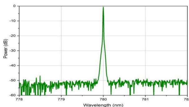
光谱(res. 10pm)
