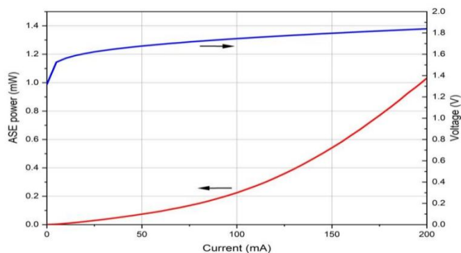
L-I-V 曲线
