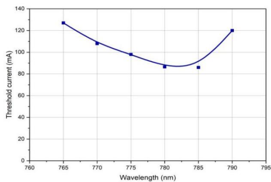
阈值电流
