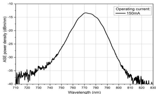
ASE 光谱 (分辨率 1nm)
