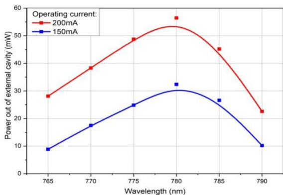
输出功率@ 780nm
