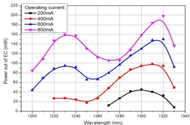
输出功率谱
