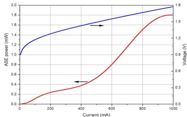
L-I-V 曲线
