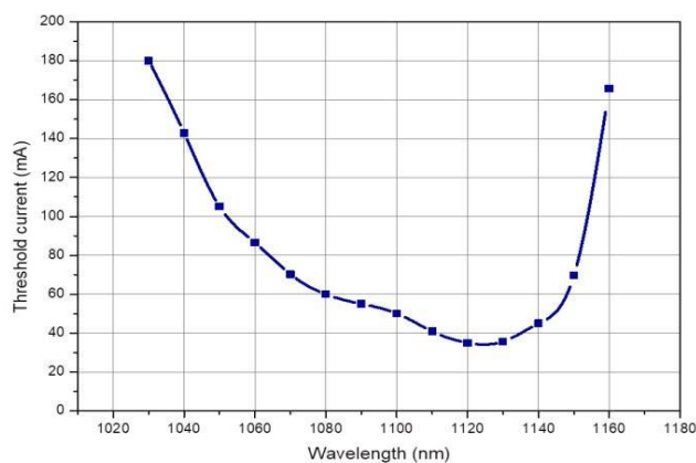
阈值电流
