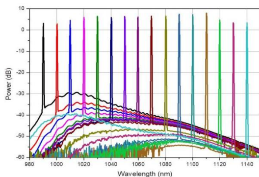
光谱(res. 0.5 nm)
