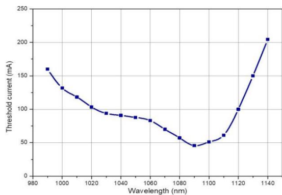
阈值电流
