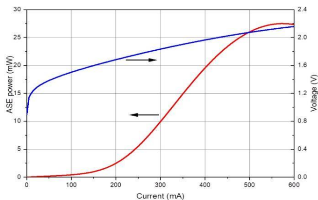
L-I-V 曲线
