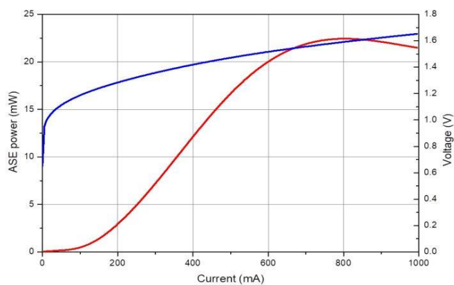
L-I-V 曲线
