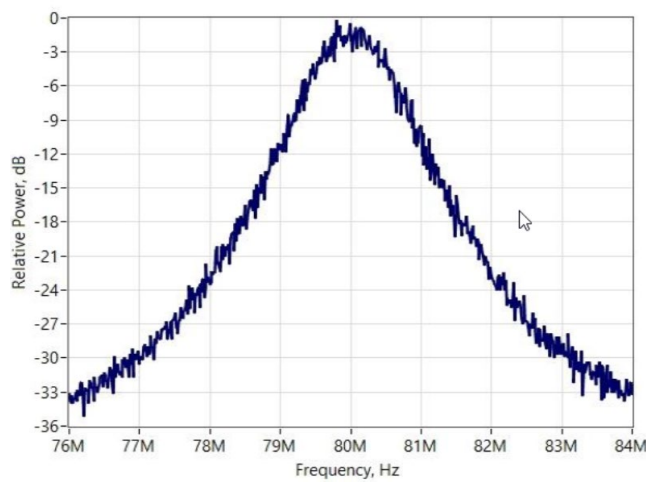
RF-line Spectrum
