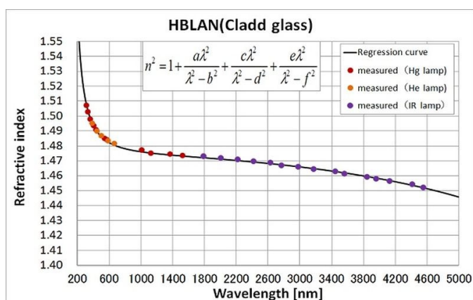
HBLAN玻璃的折射率(用于包层, 典型)
