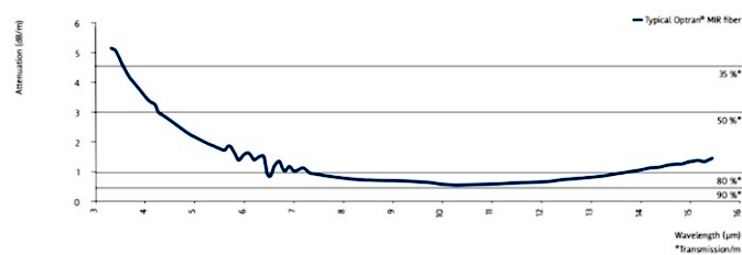
Optran® MIR
